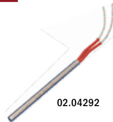
02.04292 RESISTÊNCIA PARA EXTRUSORA 220V 02.08815 SENSOR / SONDA EC SND 5100 (NTC) ● 02.04682 SENSOR / SONDA EC SND 0110 (PTC) ●
